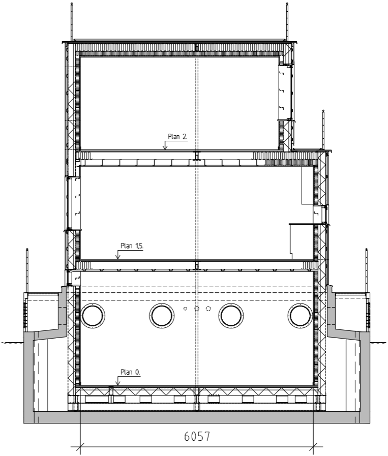
Tvärsektion, cross section
