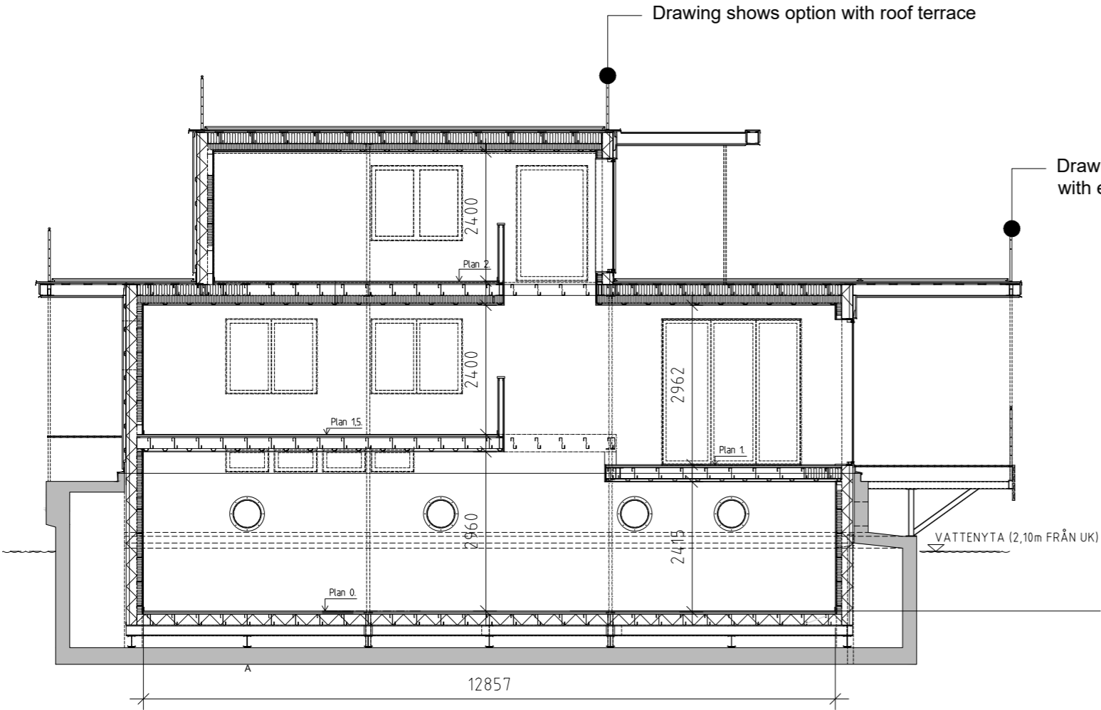
Längdsektion, longitudinal section
