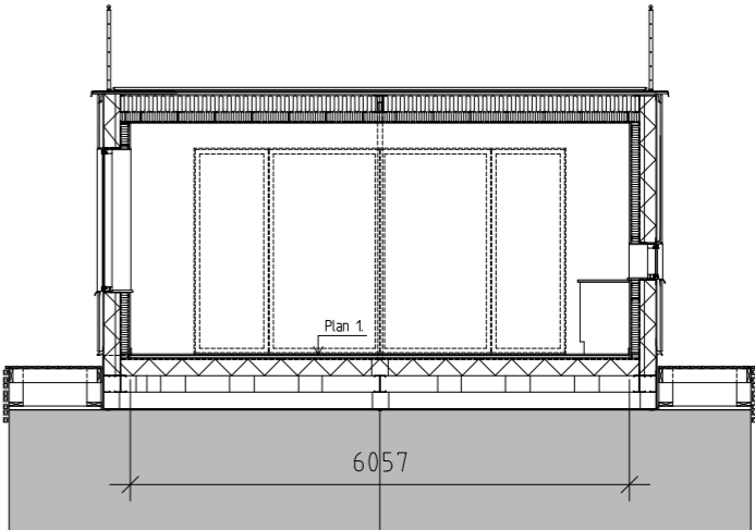
Tvärsektion, cross section
