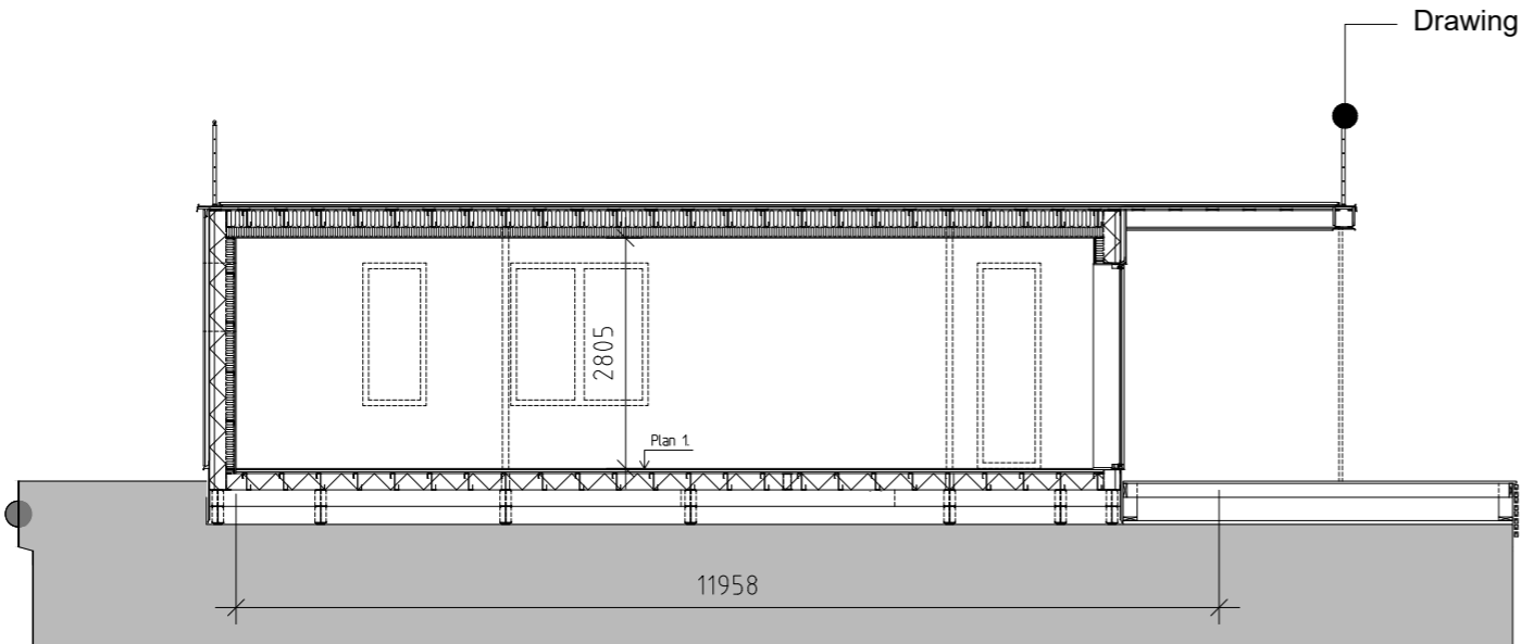
Längdsektion, longitudinal section
