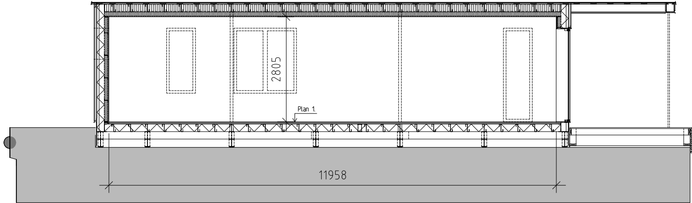
Längdsektion, longitudinal section
