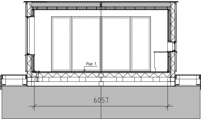
Tvärsektion, cross section
